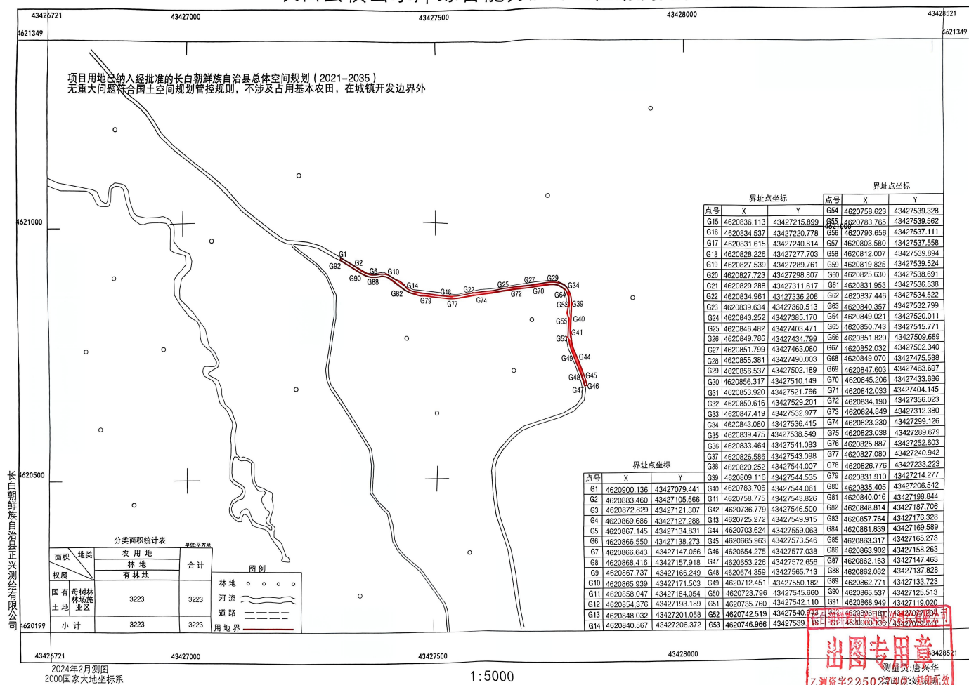
长白县横山水库综合能力提升工程勘测定界技术图4
