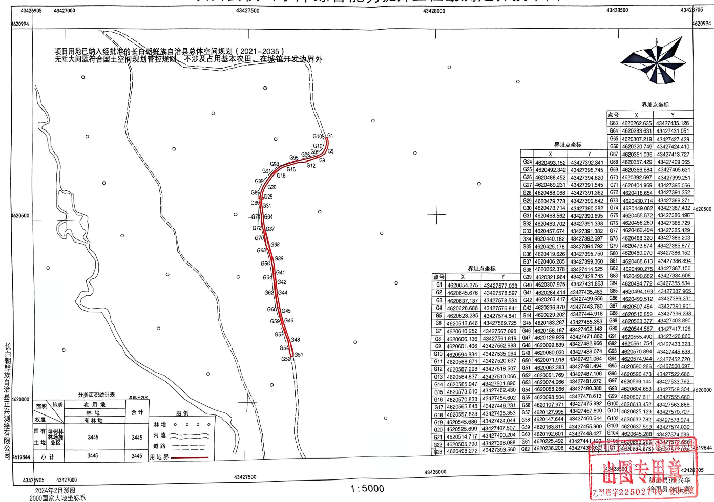
长白县横山水库综合能力提升工程勘测定界技术图5
